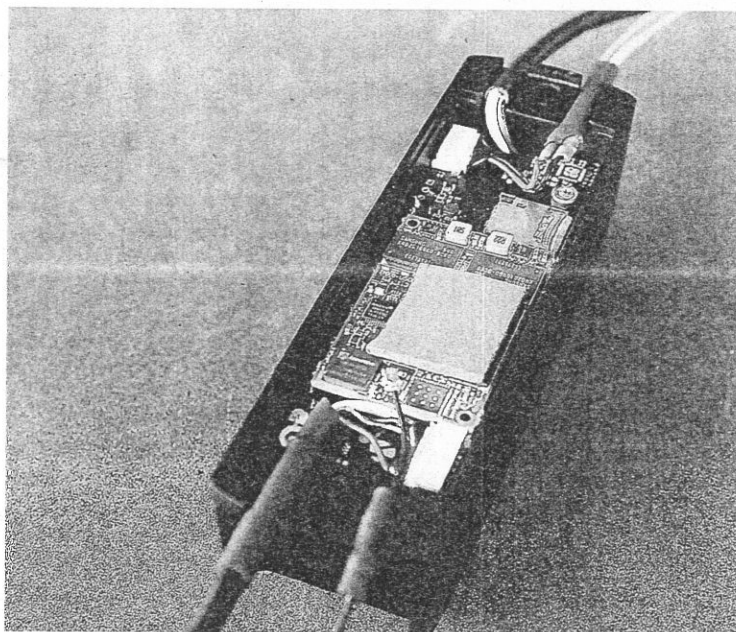
La start-up Kawantech a développé un capteur capable de distinguer un piéton, un vélo d'une automobile pour commander la puissance d'éclairage du lampadaire.
